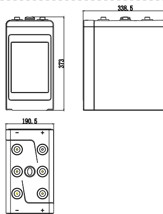
备注：所有尺寸的公差为±2mm：
